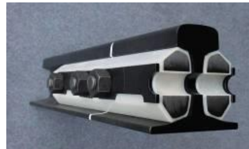
Particolare sezione giunto isolato
